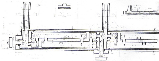
Tekening "Luftschutzkeller" (bron: NIOD)
